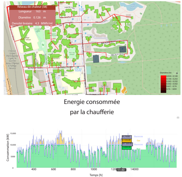
Visualisations cartographiques du tracé du réseau et consommations des moyens de production centralisés
